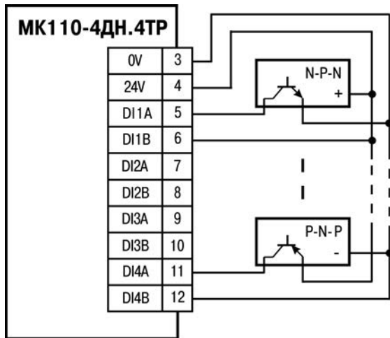
Рисунок Б.6 - Схема подключения к МК110-220.4ДН.4ТР дискретных датчиков с транзисторным выходом р-н-р-типа и н-р-п-типа с ОК (пример)
