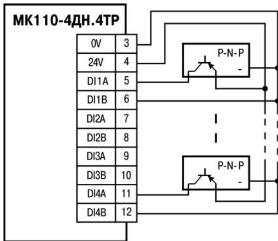
Рисунок Б.5 - Схема подключения к МК110-220.4ДН.4ТР дискретных датчиков с транзисторным выходом р-п-п-типа
