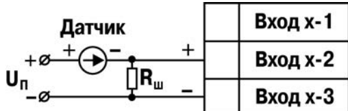
Рисунок Б.5 - Схема подключения активного датчика с токовым выходом 0...5.0, 0...20.0 или 4...20.0 мА ( R_{ш}=50,000 \pm 0,025 \text{ Ом} )
