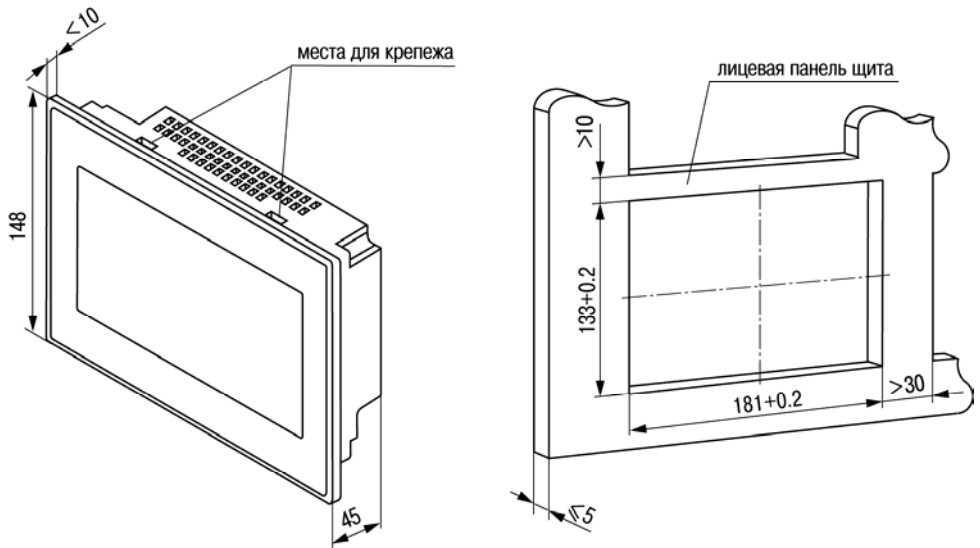
Рисунок А.2 - Установочные размеры
