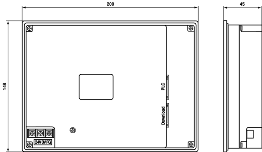
Рисунок А.1 - Габаритные размеры
