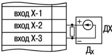
в) датчик с унифицированным выходным сигналом тока
