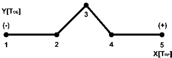
Рисунок 5.4 – Пример графика температуры обратной воды
