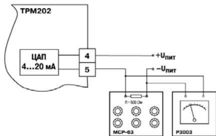
Рисунок Ж.4 – Подключение ВУ1 типа И ( R_H=500 \text{ Ом} )
