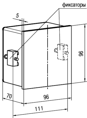
Рисунок А.3 – Прибор щитового крепления Щ1
