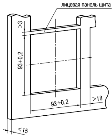
Рисунок А.3 – Прибор щитового крепления Щ1
