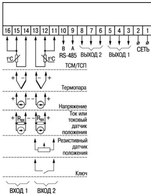
Рисунок Б.2 – Общая схема подключения TRM212-H2
