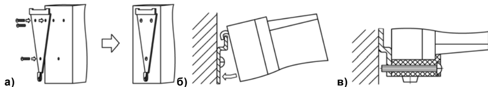
Рисунок 5.1 Монтаж прибора настенного исполнения Н
