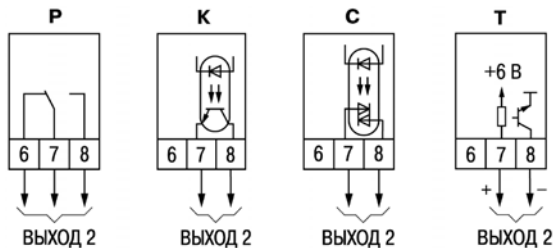
Рисунок Б.4 – Схемы подключения к различным типам ВУ2
