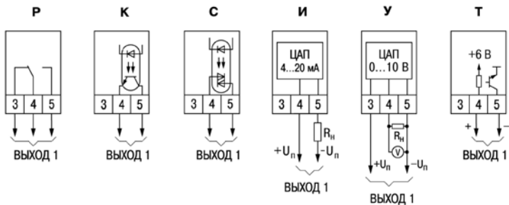
Рисунок Б.3 – Схемы подключения к различным типам ВУ1
