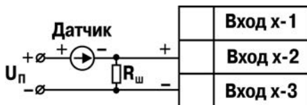
Рисунок Б.6 – Подключение активного датчика с токовым выходом 0...5 мА или 0(4)...20 мА ( R_{ш} = 100,0 \text{ Ом} \pm 0,1\% )
