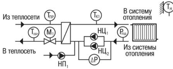
Рисунок Л.1 - Одноконтурная система отопления с циркуляционными насосами и насосом подпитки
