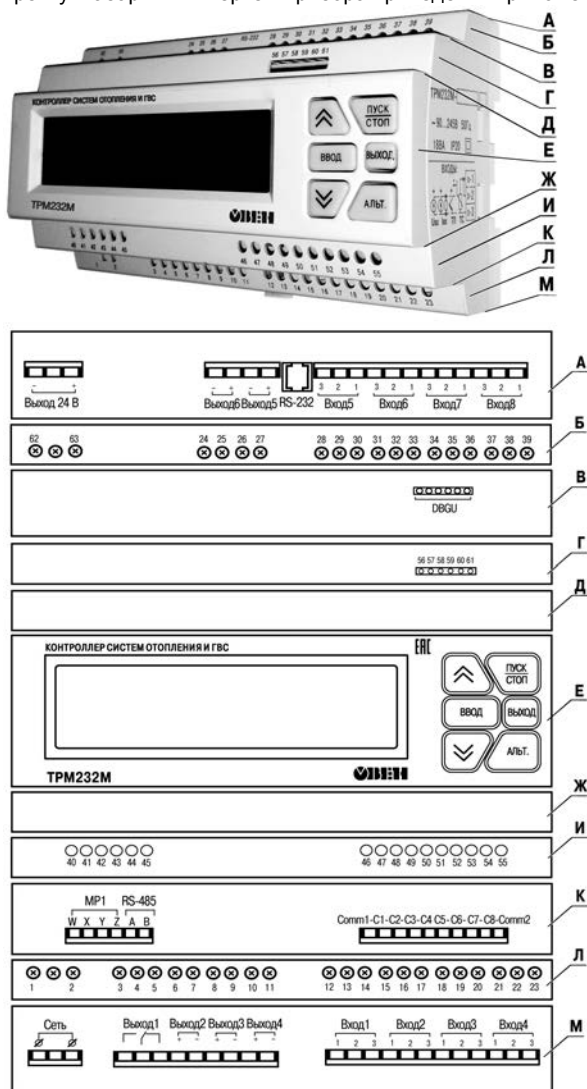
Рисунок 3.1 – Прибор TRM232M: клеммники, элементы индикации и управления
