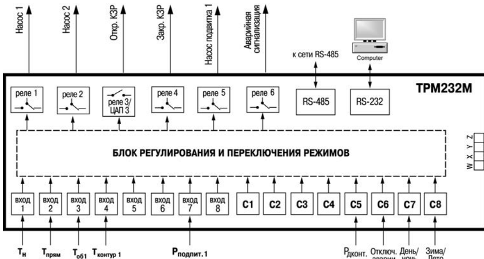
Рисунок 3.8 – Функциональная схема прибора, один контур
