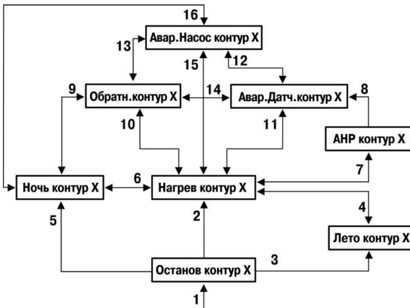
Рисунок 4.2 – Схема перехода между режимами контура
