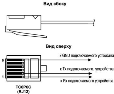
Рисунок Д.3 – Схема распыки соединительного кабеля для подключения к порту RS-232
