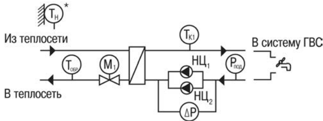
Рисунок Л.2 - Одноконтурная система ГВС с циркуляционными насосами и насосом подпитки
