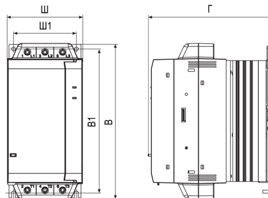
Рисунок 1 – Габаритные размеры
