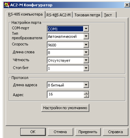
Рисунок 9.1 – Конфигуратор AC2-M. Вкладка «RS-485»
