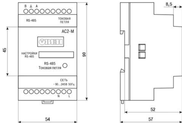
Рисунок А.1 - Габаритный чертеж преобразователя АС2-М
