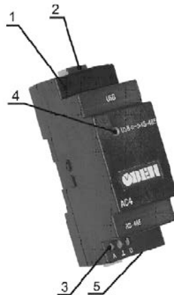
Рисунок 4.1 – Внешний вид прибора AC4
