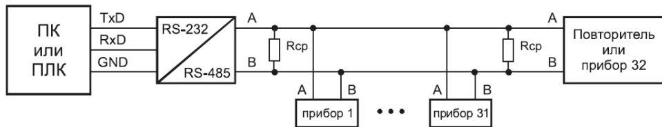
Рисунок 1.1 – Типовая топология промышленной сети RS-485
