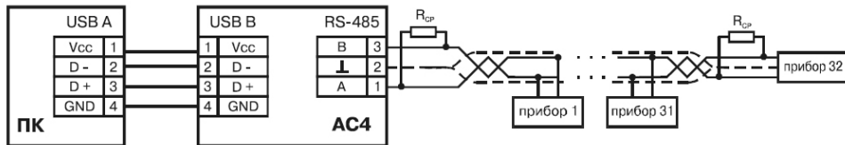
Рисунок 6.1 – Схема подключения прибора AC4
