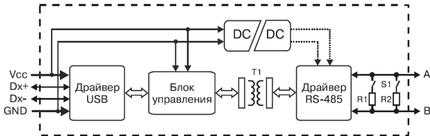
Рисунок 4.2 – Функциональная схема прибора AC4
