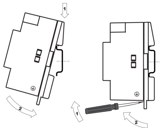
Рисунок 2 – Монтаж (а) и демонтаж (б) прибора
