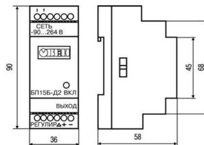
Рисунок 3.1 – Габаритные размеры блока питания БП15Б-Д2-х
