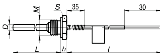
Рисунок А.3 – Конструктивное исполнение 054, 064, 074 и 194
