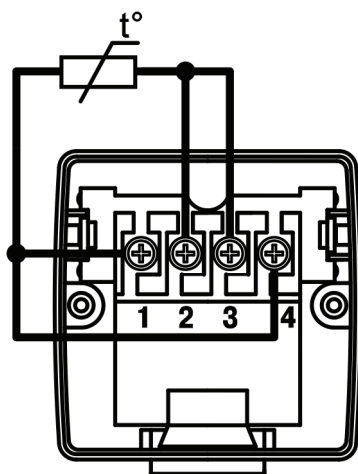
в) четырехпроводная
