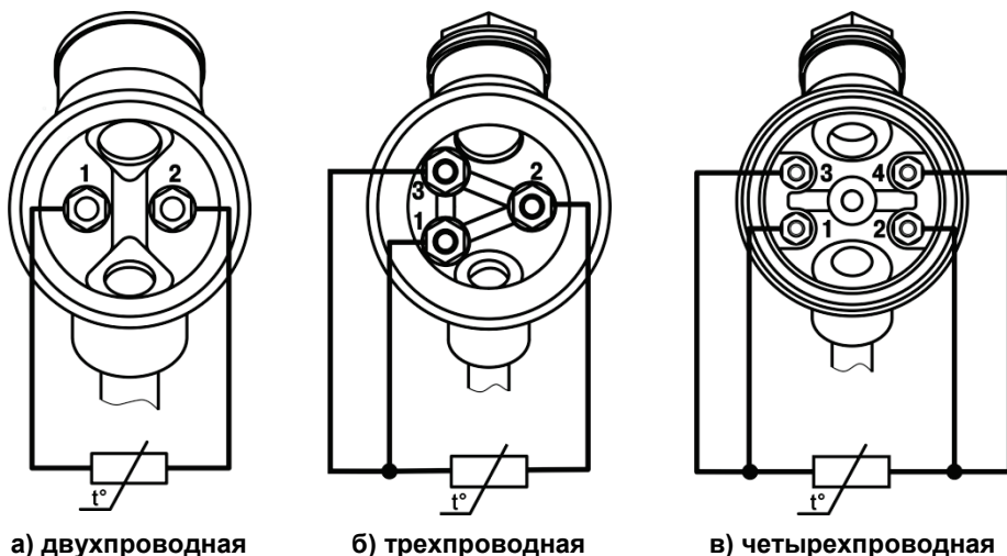
Рисунок Е.1 – Схемы подключения проводов к клеммам пластмассовых коммутационных головок датчиков типа ДТС ХХ5 с одним ЧЭ
