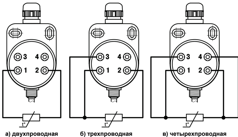
Рисунок Е.3 – Схемы подключения проводов к клеммам пластмассовых коммутационных головок датчиков типа ДТС 125Л с одним ЧЭ
