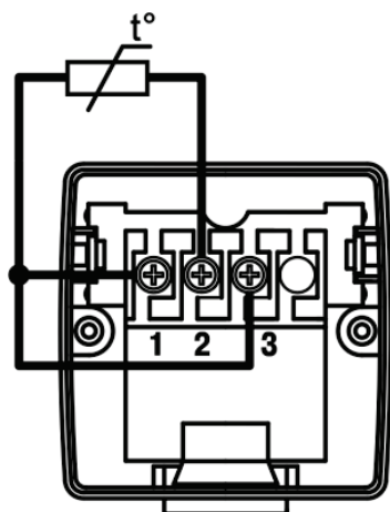
б) трехпроводная
