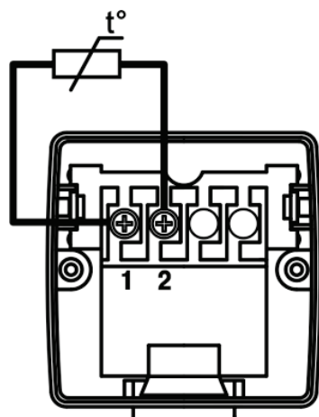
а) двухпроводная
