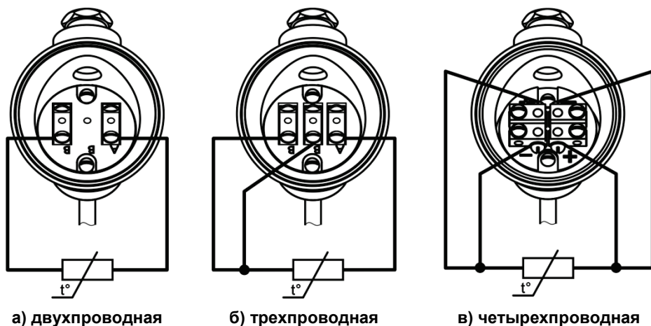
Рисунок Е.2 – Схемы подключения проводов к клеммам металлических коммутационных головок датчиков типа ДТС ХХ5 с одним ЧЭ
