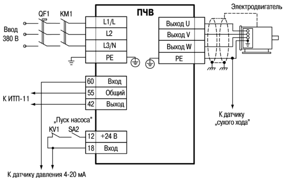
Рисунок Б.1 – Схема подключений
